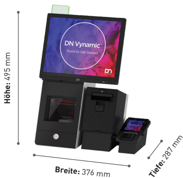
Tischmontage Höhe: 495 mm Breite: 376 mm Tiefe: 287 mm
