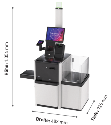
Cash Rack-Montage Höhe: 1.354 mm Breite: 483 mm Tiefe: 720 mm
