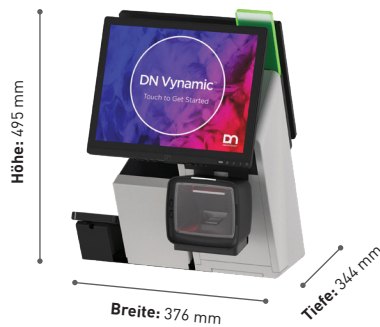
Assisted-Service-Variante Höhe: 495 mm Breite: 376 mm Tiefe: 344 mm
